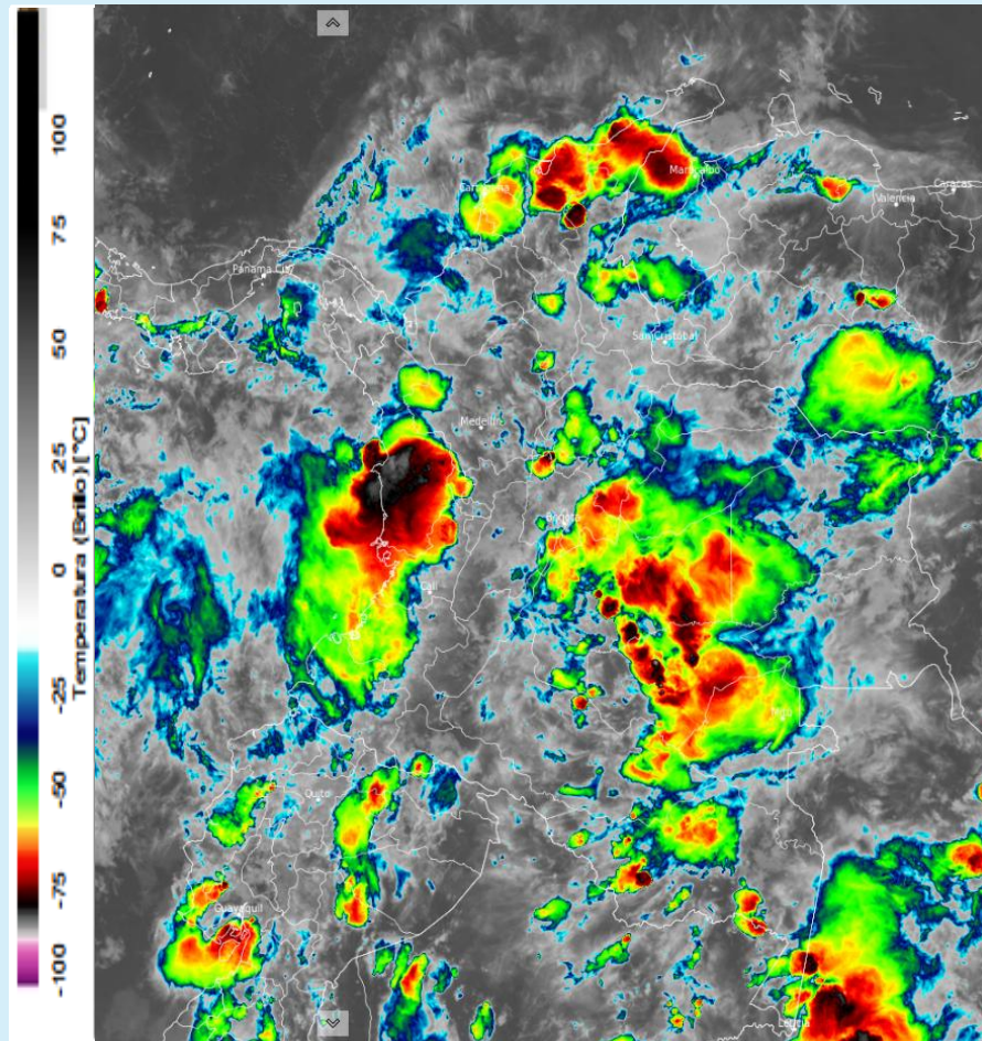
Imagen GOES 19 (East) Canal Infrarrojo 10 de abril de 2025 - Hora 17:30 HLC Fuente: Rammslider
