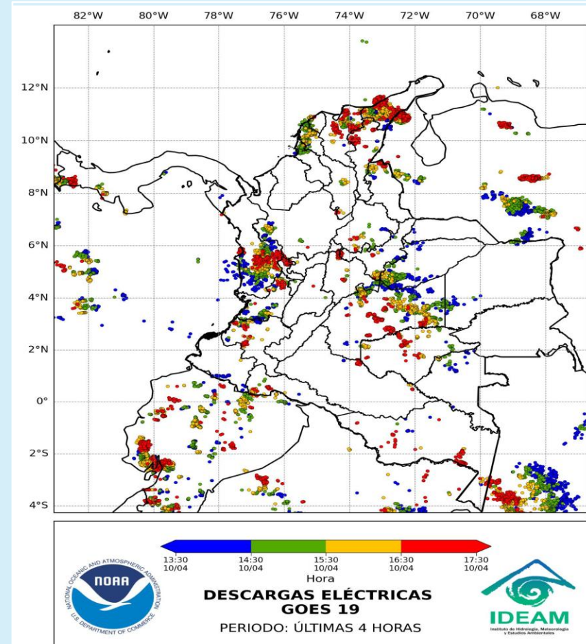
Descargas eléctricas últimas 4 horas 10 de abril de 2025 - Hora 17:30 HLC Fuente: IDEAM
