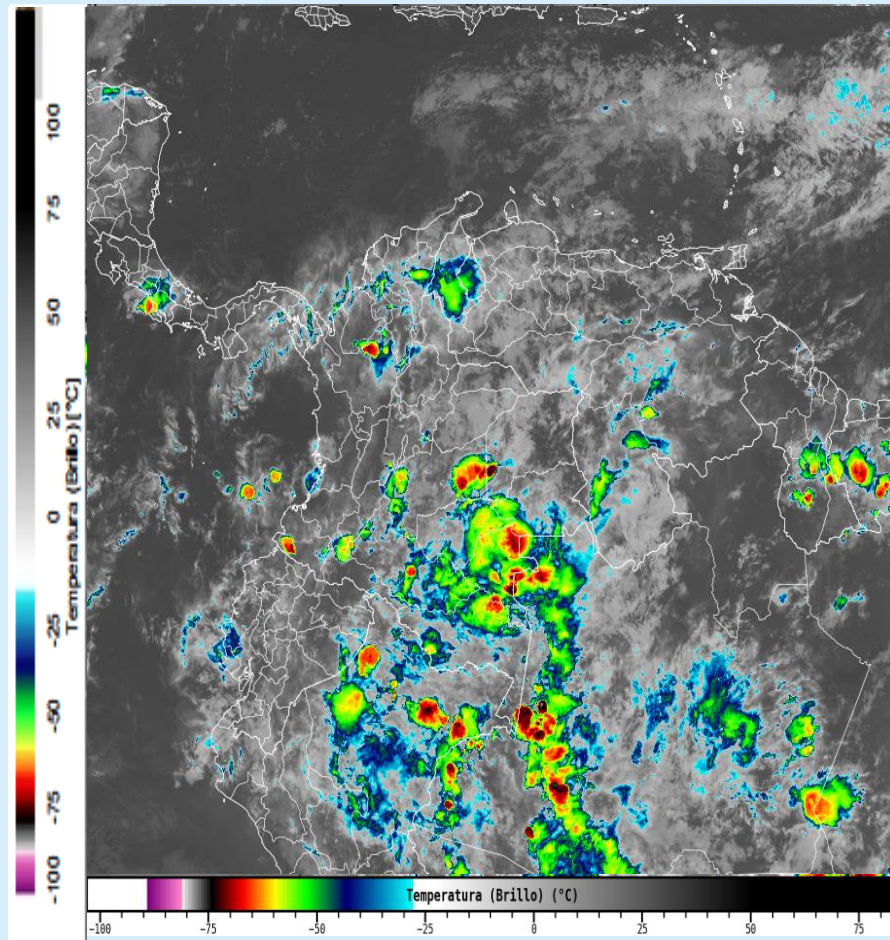
Imagen GOES 19 (East) Canal Infrarrojo 8 de abril de 2025 - Hora 23:10 HLC Fuente: IDEAM
