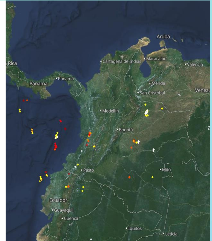
Descargas eléctricas en las últimas cuatro horas. Fuente: map.blitzortung.org
