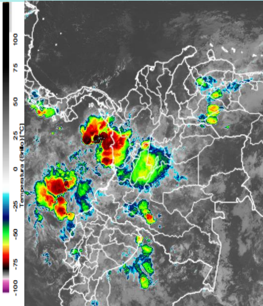
Imagen GOES East Canal Infrarrojo, 8 de abril de 2025 - Hora 11:30 HLC. Fuente: rammb-slider.cira.colostate.edu
