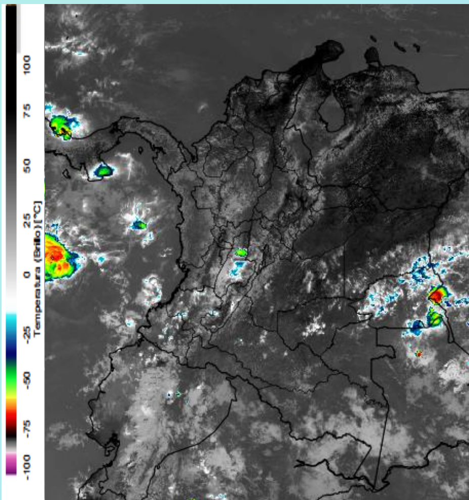
Imagen GOES East Canal Infrarrojo, 25 de abril de 2020. Hora 11:40 HLC. Fuente: IDEAM-GOES 16
