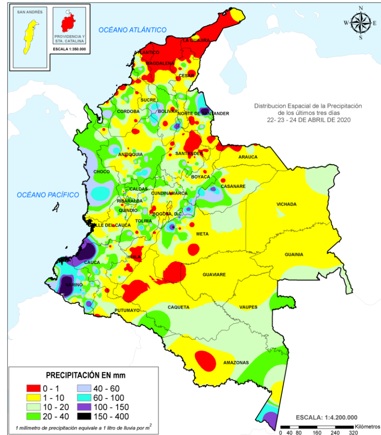
Precipitación últimas 72 horas desde las 7:00 HLC del miércoles 22 de abril hasta las 7:00 HLC del sábado, 25 de abril de 2020. Fuente: IDEAM
