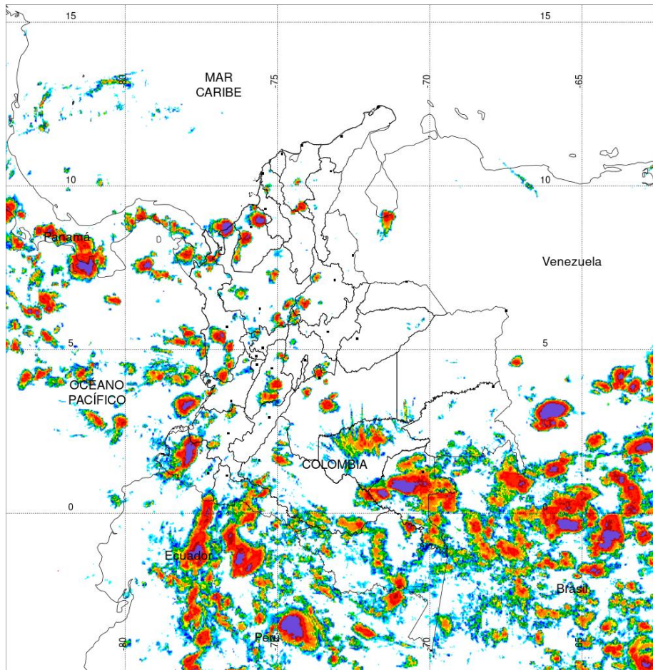
PRECIPITACIÓN TOTAL ACUMULADA POR ESTIMACIÓN SATELITAL (GOES-16) APR 24 DE 2020 (7:00) - APR 25 DE 2020 (7:00)
