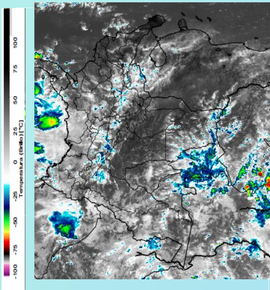
Imagen GOES East Canal Infrarrojo 7 de diciembre de 2019. Hora 11:20 HLC. Fuente: IDEAM-GOES 16
