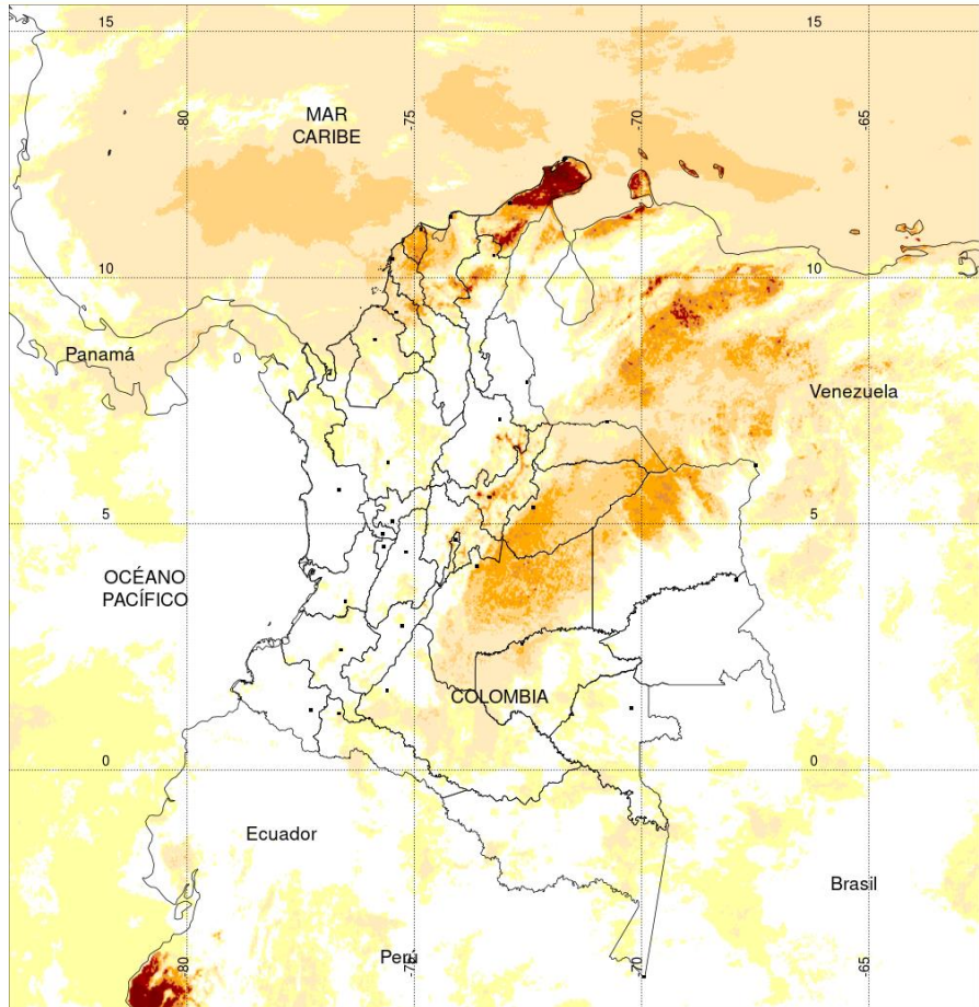
TEMPERATURA SUPERFICIAL MÁXIMA POR ESTIMACIÓN SATELITAL (GOES-16) ( 2019-12-07 09:00:00 a 2019-12-07 11:10:00 )
