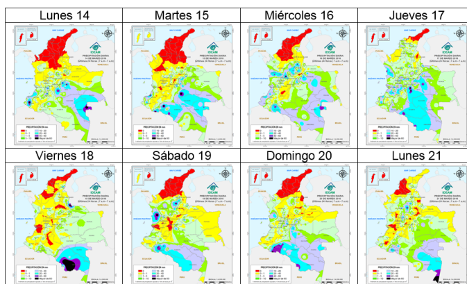
Figura 1: Precipitación diaria del lunes 14 al lunes 21 de marzo de 2016. Fuente: Grupo de datos - IDEAM
